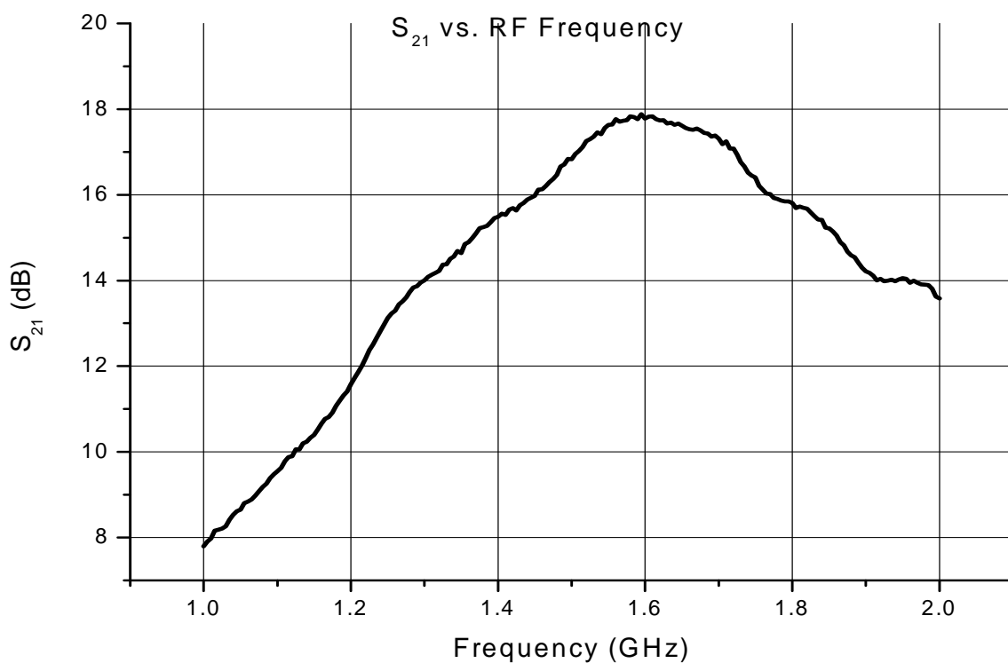
图四、功率增益与工作频率的曲线
