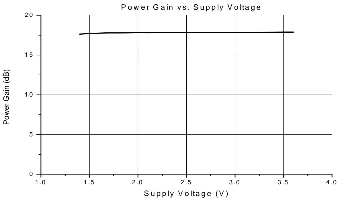
图三、功率增益与供电电压的曲线
