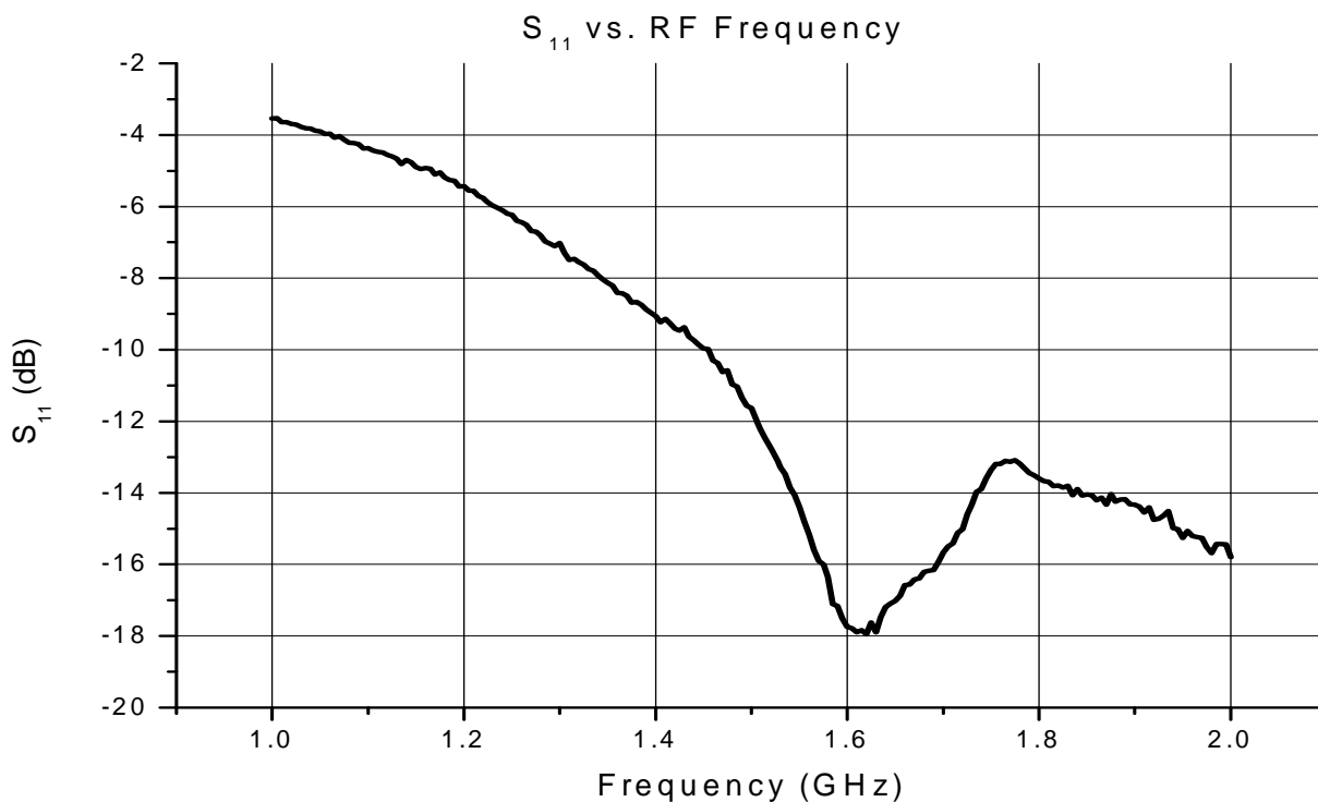
图五、输入回损与工作频率的曲线
